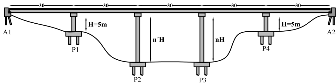
ج) پروفیل طولی پل‌ها شکل ۱. شکل نامنظمی پل‌ها
