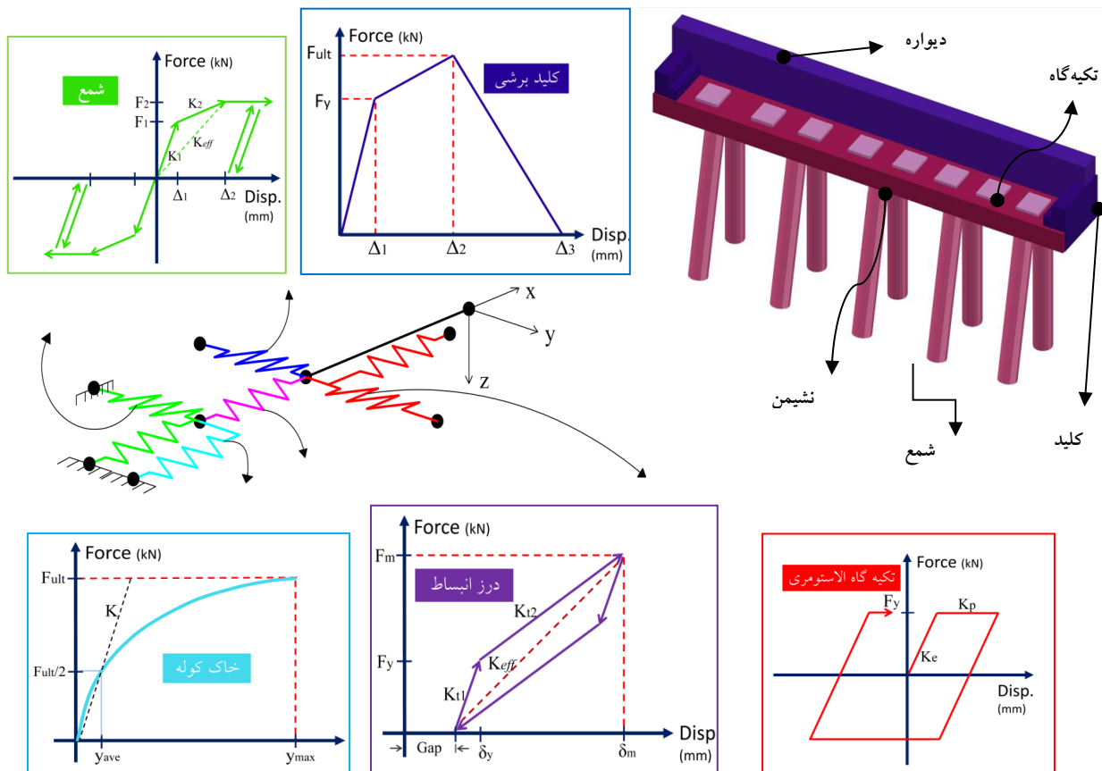
شکل ۲. شماتیک اعضای کوله، رفتار مصالح و چیدمان المان‌های آن در مدل اجزای محدود
