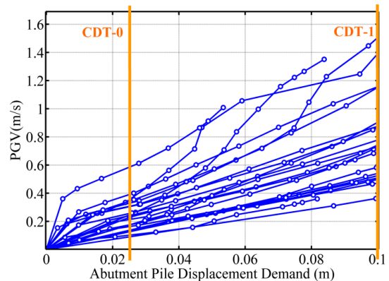
شکل ۳. نمودار IDA مربوط به تغییر مکان شمع کوله
