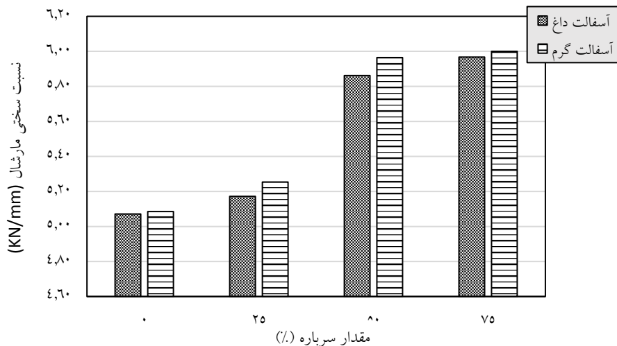
شکل ۶. نسبت سختی مارشال برای مخلوط های آسفالتی گرم و داغ
