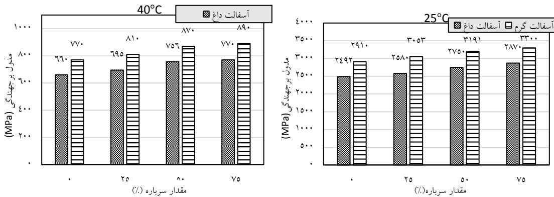
شکل ۸. مدول برجهندگی مخلوط‌های آسفالتی داغ و گرم در دماهای ۲۵ و ۴۰ درجه سلسیوس
