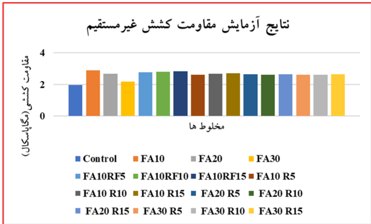
شکل ۱۲. نتایج مقاومت کششی غیرمستقیم
