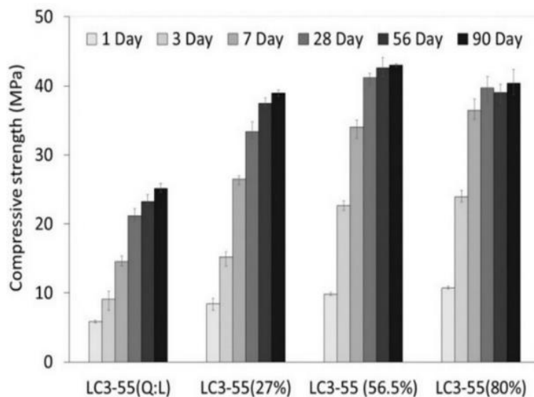
شکل ۴. تأثیر محتوای کائولینیت خاک رس کلسینه‌شده (۲۷٪، ۵۶٪/۵ و ۸۰٪) بر مقاومت فشاری (کریشان و بیشنوی، ۲۰۲۰)
