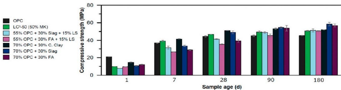
شکل ۵. مقایسه مقاومت فشاری سیمان LC3 با دیگر سیمان‌ها (زونیو و اسکینور، ۲۰۲۱)
