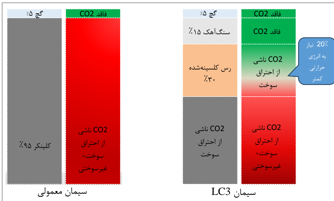
شکل ۲. مقایسه ترکیب سیمان پرتلند معمولی و سیمان LC3 (باربوتیا و همکاران، ۲۰۲۳)
