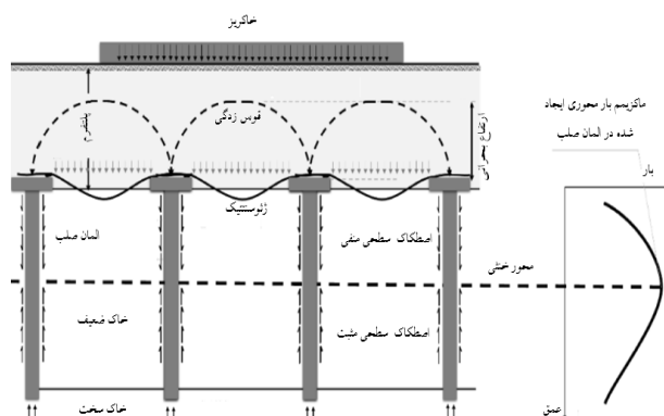
شکل ۵. مکانیزم خاگریز مسلح شده با ژئوسنتتیک و متکی بر المان صلب (ربولدو و کارالو، ۲۰۱۹)
