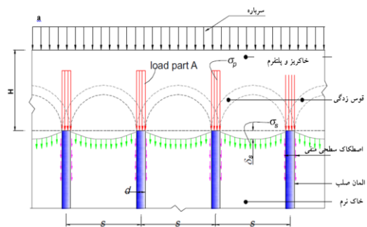
شکل ۸ مکانیسم انتقال بار، a: خاکریز متکی بر شمع و b: خاکریز مسلح شده با ژئوسنتتیک و شمع (فام، ۲۰۱۸)
