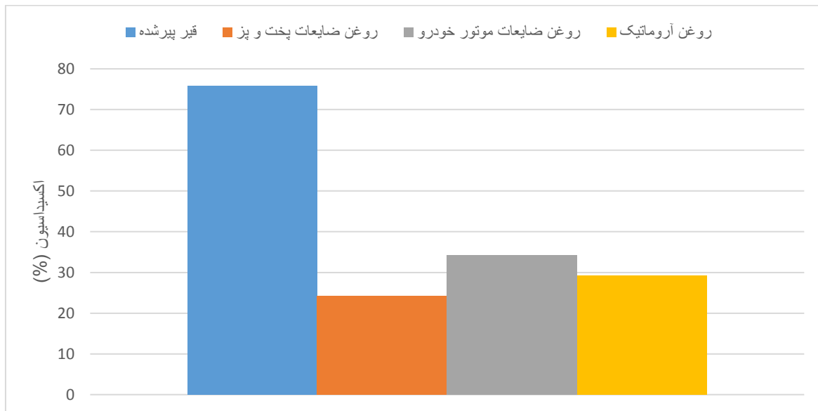
شکل ۷. تأثیر انواع جوانسازها بر اصلاح درصد اسیدیته
