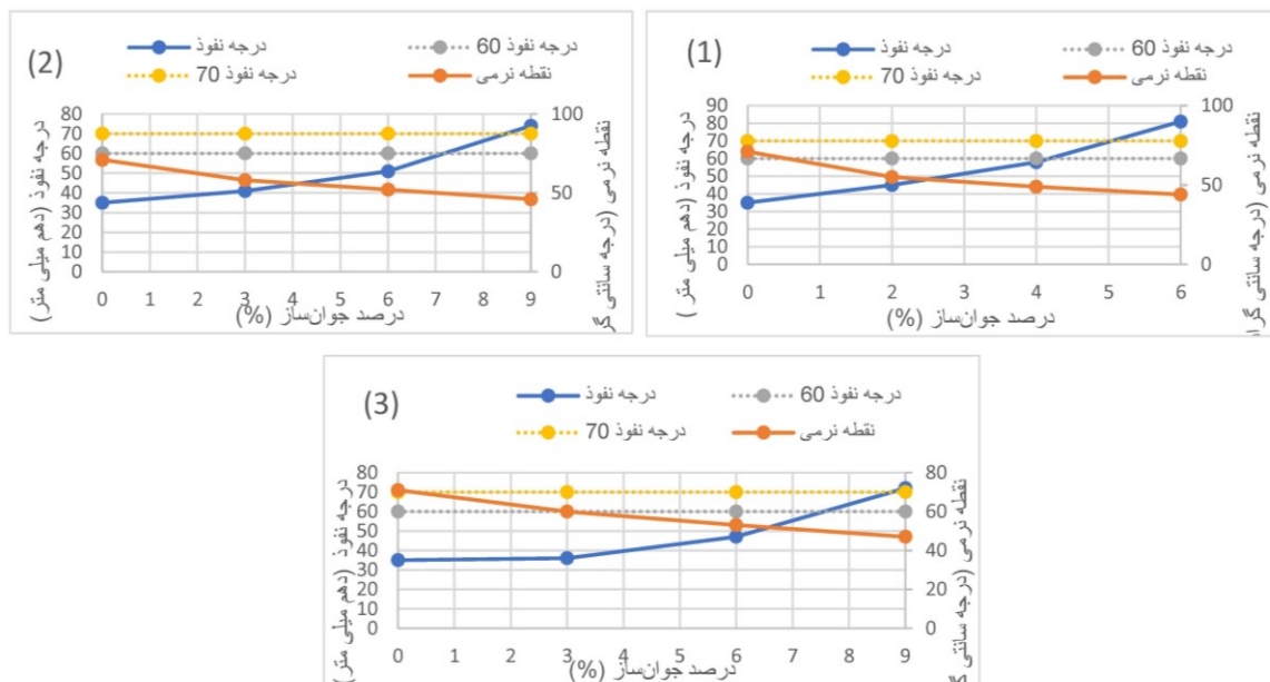
شکل ۱. مقادیر درجه نفوذ و نقطه نرمی در درصدهای مختلف: (۱) روغن ضایعات پخت‌وپز، (۲) روغن ضایعات موتور و (۳) روغن آروماتیک
