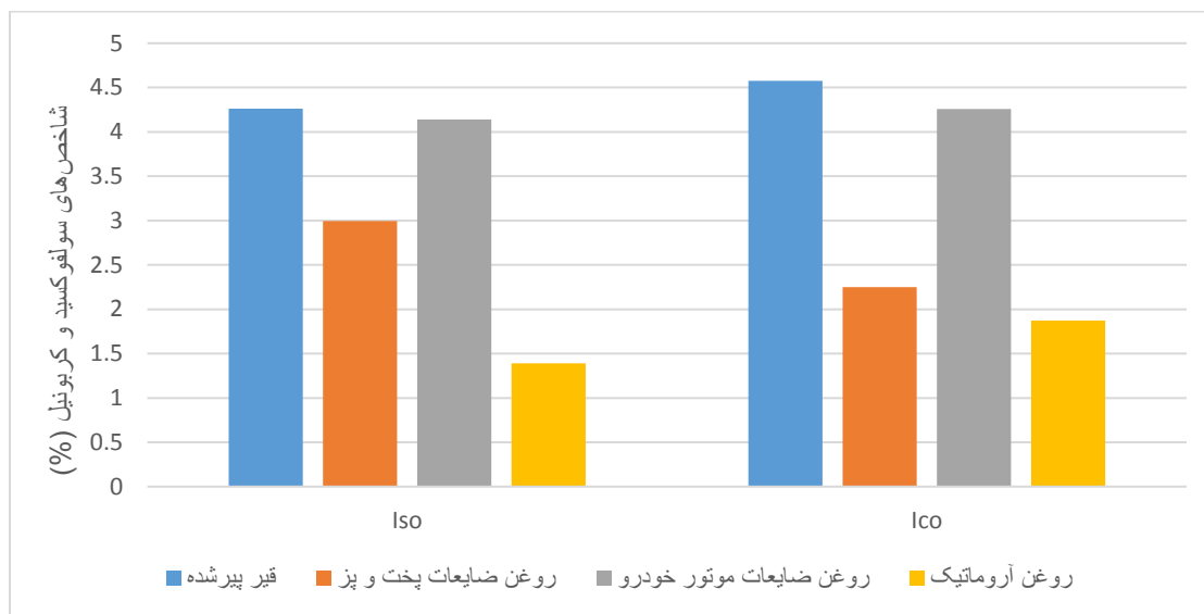
شکل ۵. تأثیر انواع جوان‌سازها بر اصلاح شاخص‌های سولفوکسید و کربونیل
