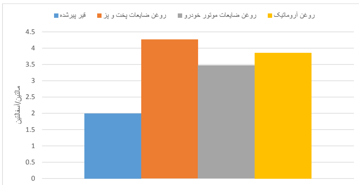
شکل ۶. تأثیر جوان‌سازهای متفاوت بر اصلاح نسبت مالین به آسفالتین
