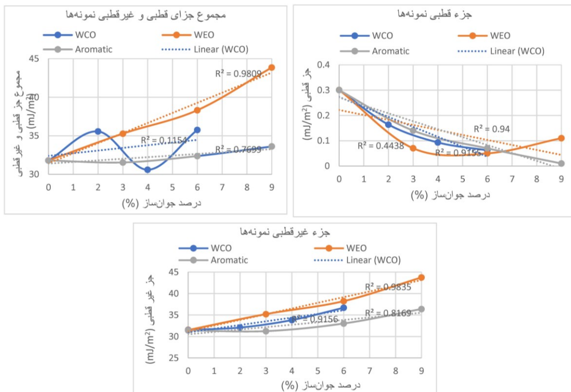
شکل ۲. تأثیر افزایش درصد جوان‌ساز بر تغییرات اجزای قطبی و غیرقطبی آزمایش انرژی آزاد سطح
