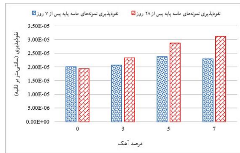
شکل ۱۷. تغییرات نفوذپذیری نمونه‌های ماسه پایه، پای، ۷ و ۲۸ روز
