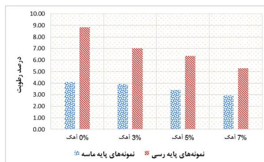
شکل ۱۰. تغییرات PI طی تثبیت خاک
