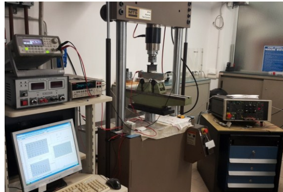
شکل ۵. انجام آزمایش تیرچه خمشی سه نقطه ای
